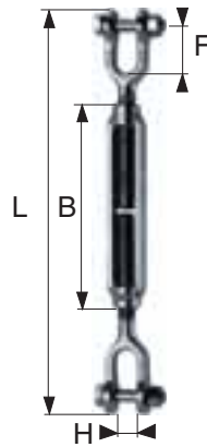
réf 5322 2 chapes
