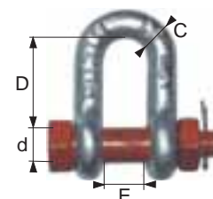
Réf 5221 : axe boulonné
