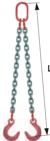
2 crochets de fonderie
