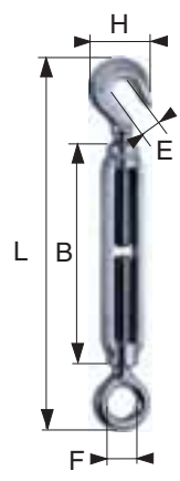
réf 5327 1 croc, 1 oeil rond
