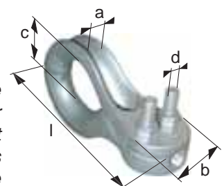
Modèle avec évidement (codes D à L)
