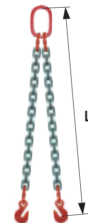
2 crochets raccourcisseurs
