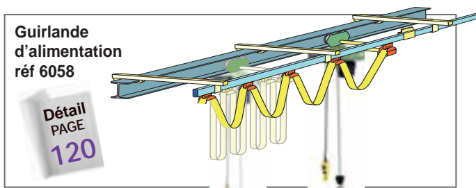
TYPE CS Suspente par chariot libre
