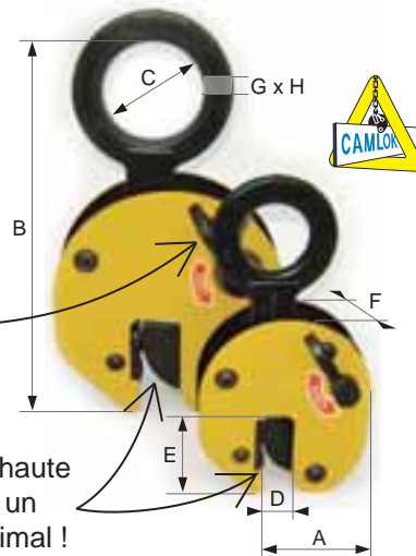
utiliser 2 pinces avec un palonnier
